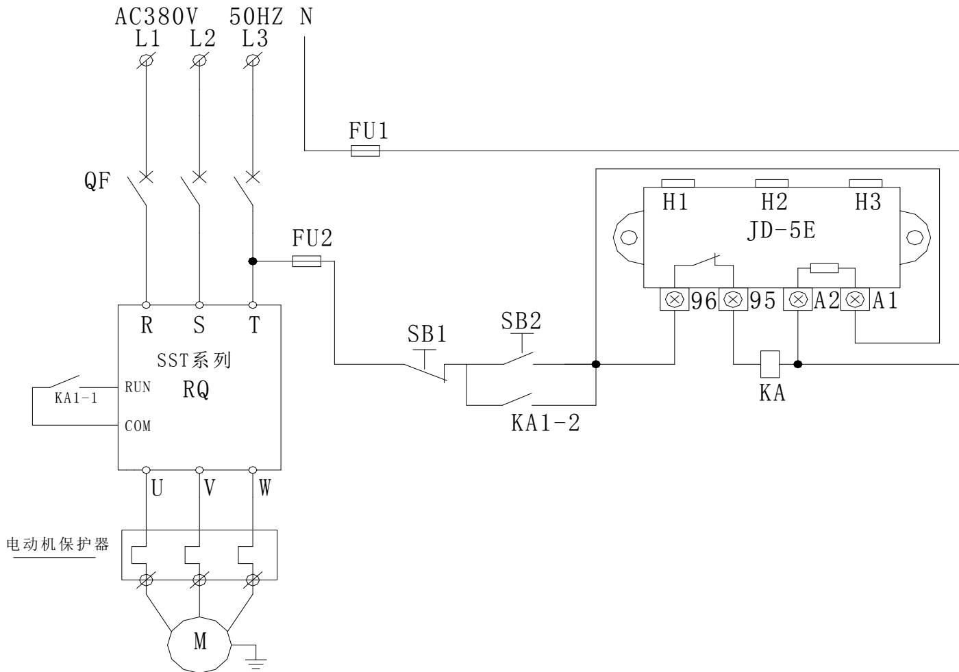
保护器与软起动器接线图 图 1
